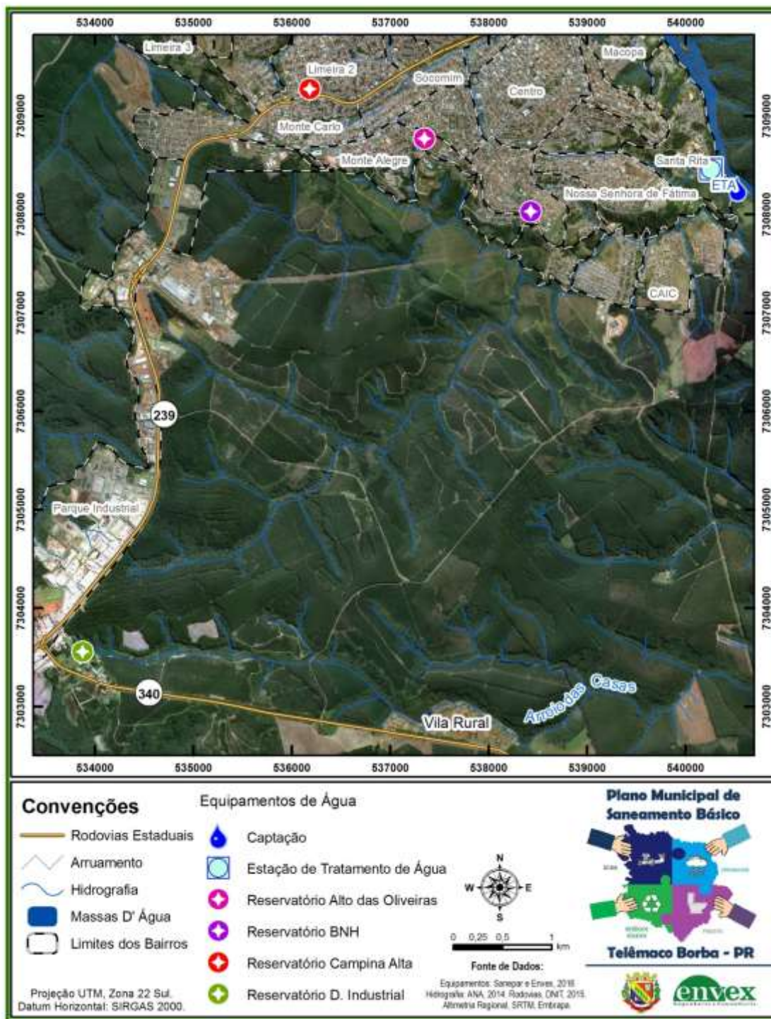
Figura 50: Localização dos componentes do sistema de abastecimento de água da área urbana de Telêmaco Borba.
