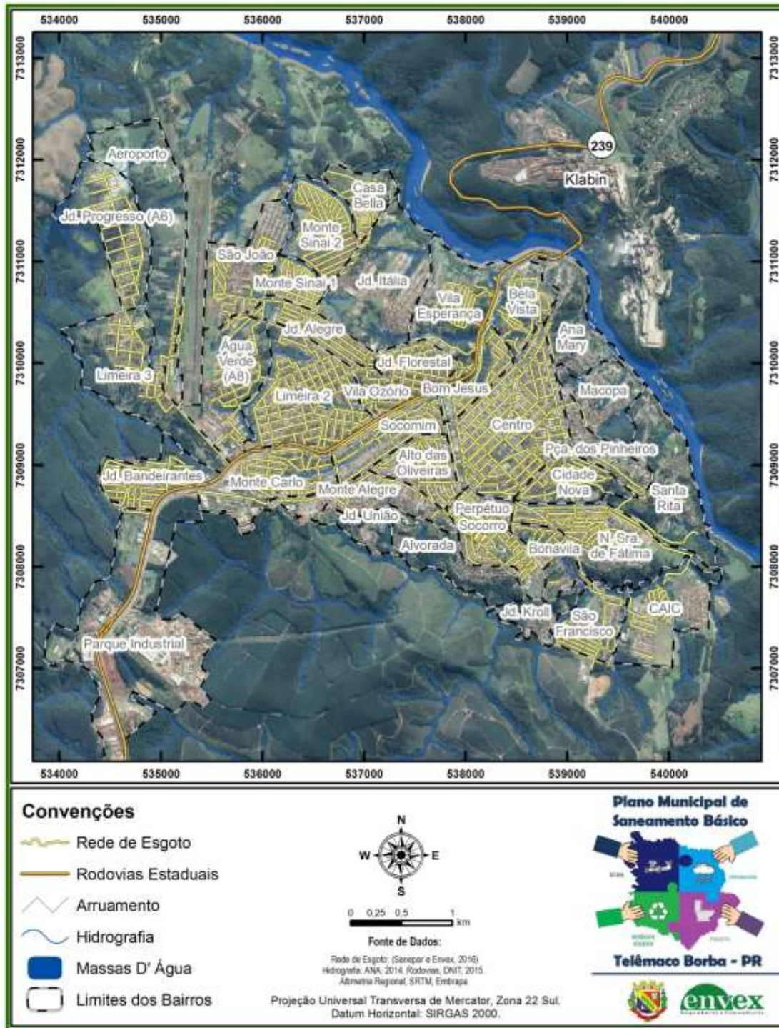
Figura 75: Rede coletora do sistema de esgotamento sanitário de Telêmaco Borba.
